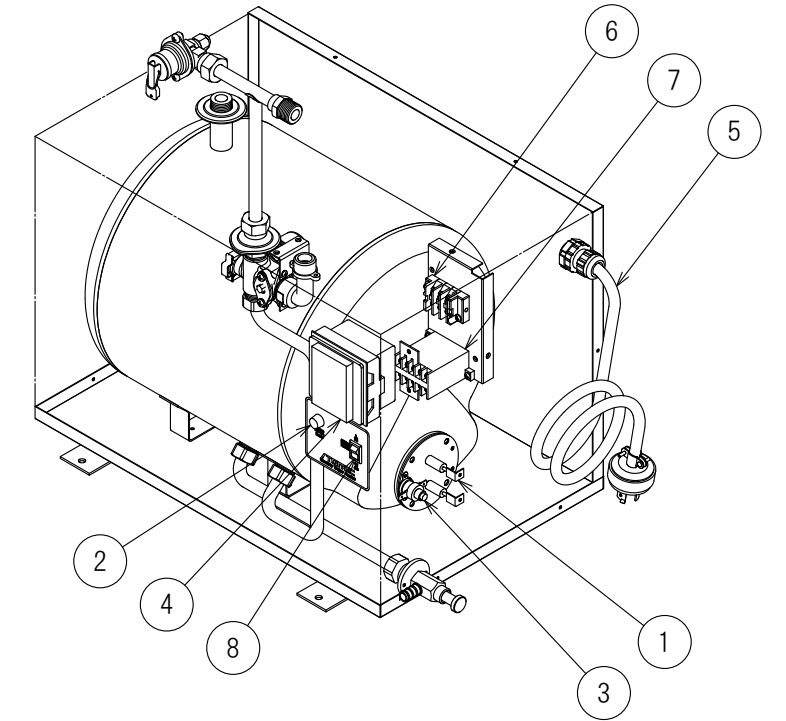
部品配置図
