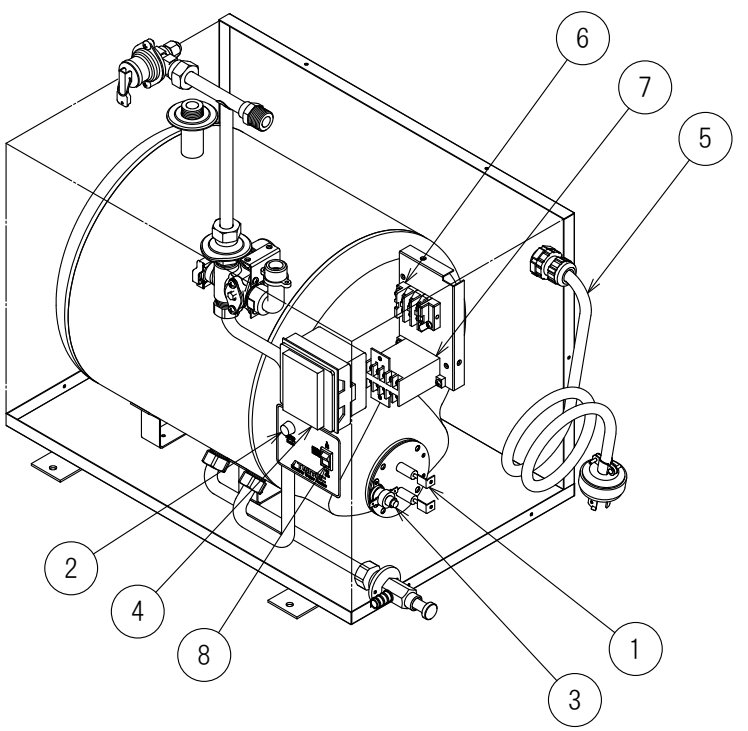
部品配置図
