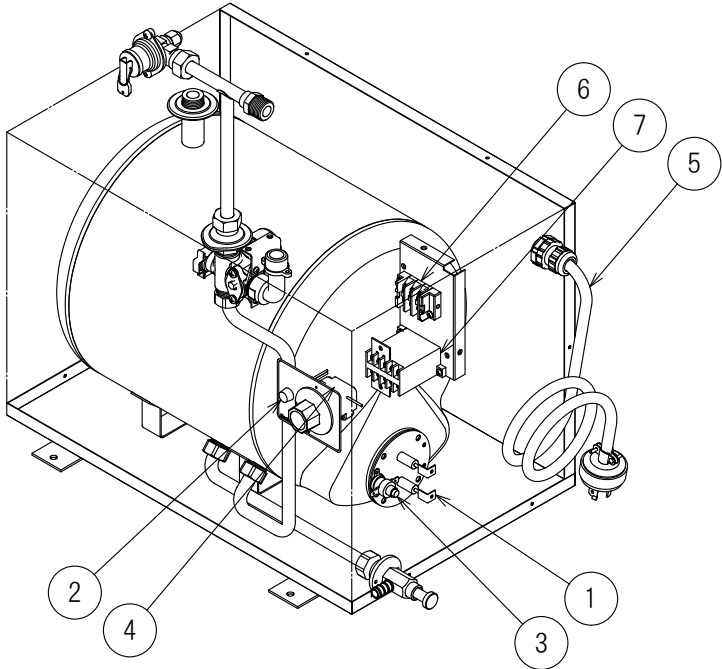
部品配置図
