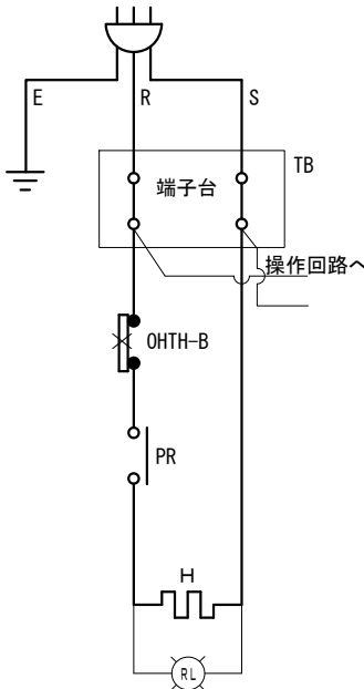
② 単相
