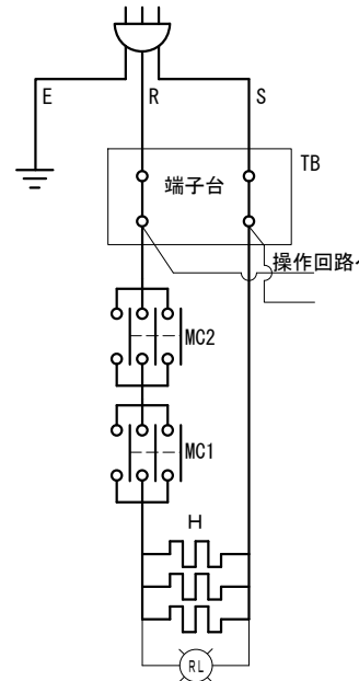
④ 単相
