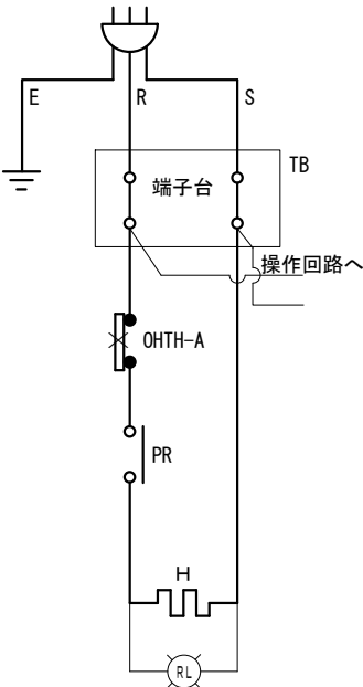
① 単相
