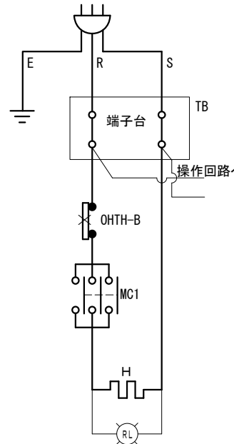
③ 単相
