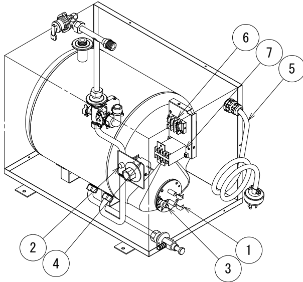
部品配置図
