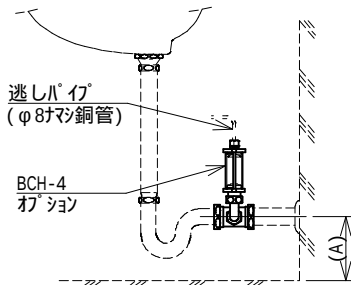
ブローキャッチャー ( BCH-4 ) 取付け例
