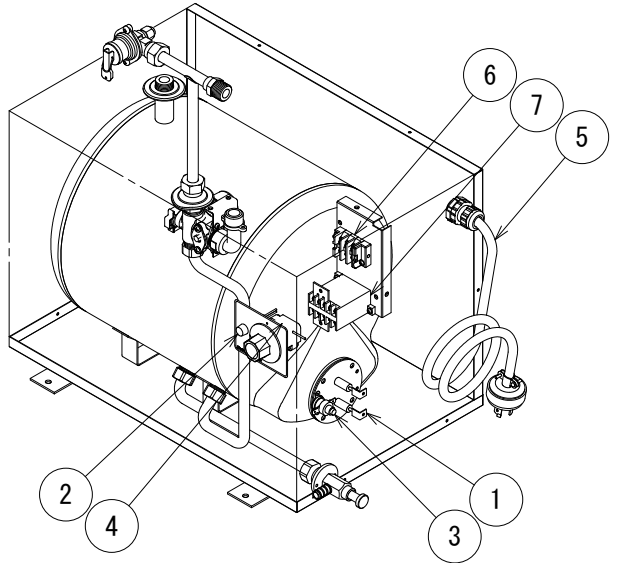
部品配置図
