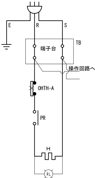
① 単相
