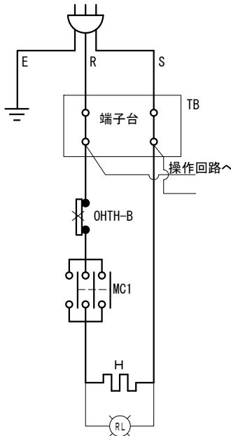
③ 単相
