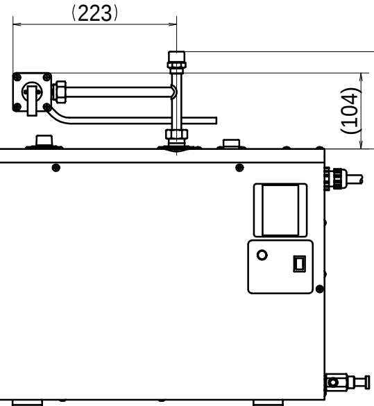
袋ナットチーzの取り付けを 変えた場合の逃し弁高さ 注7
