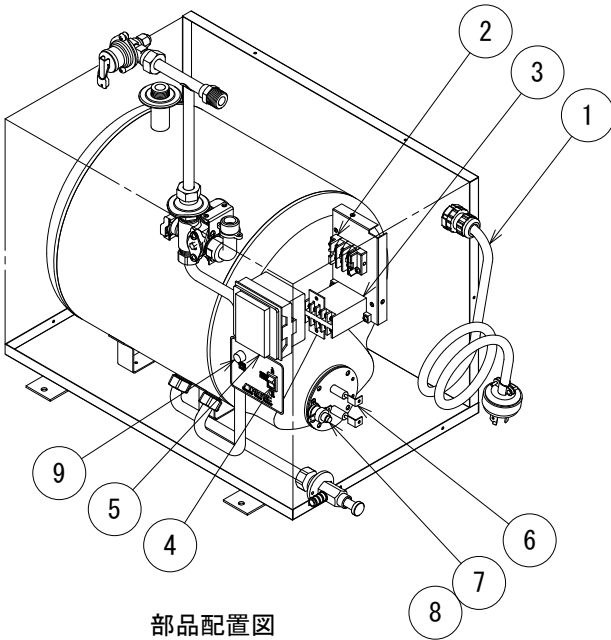
部品配置図
