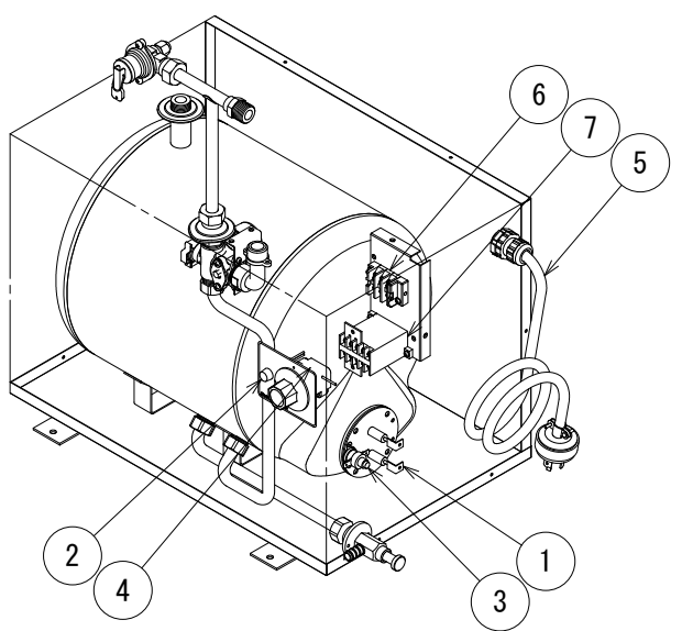
部品配置図
