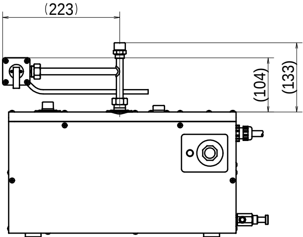
袋ナットチーズの取付けを 変えた場合の逃し弁高さ 注7
