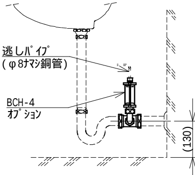
ブローキャッチャー（BCH-4）取付け例
