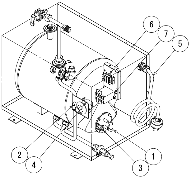
部品配置図
