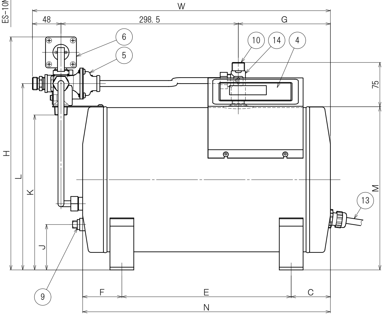
正面図
