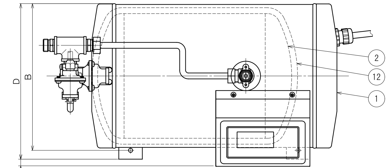
平面図
