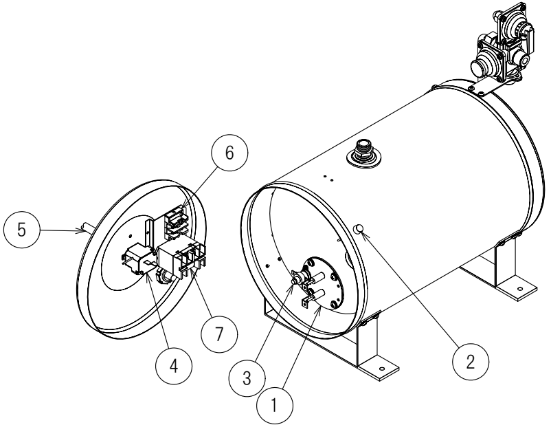
部品配置図
