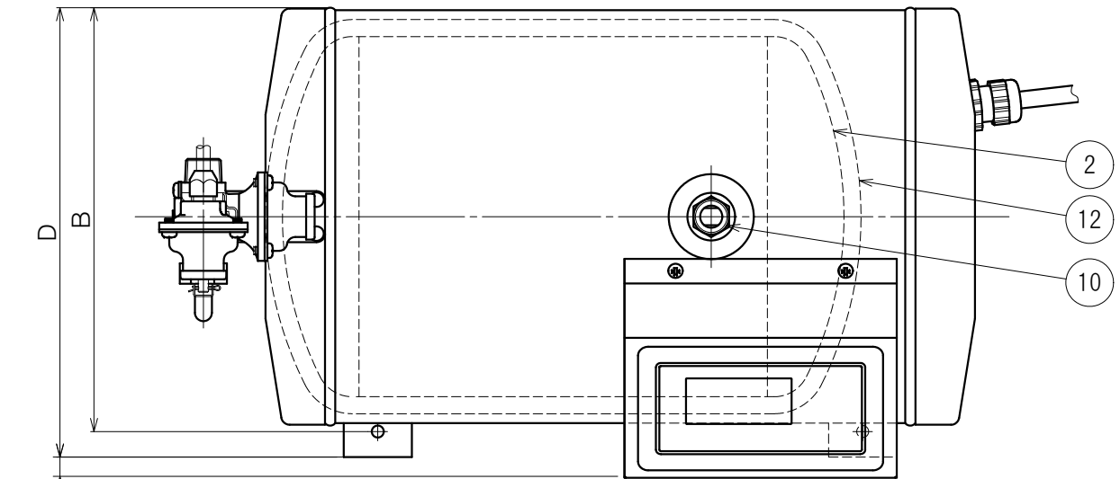
平面図
