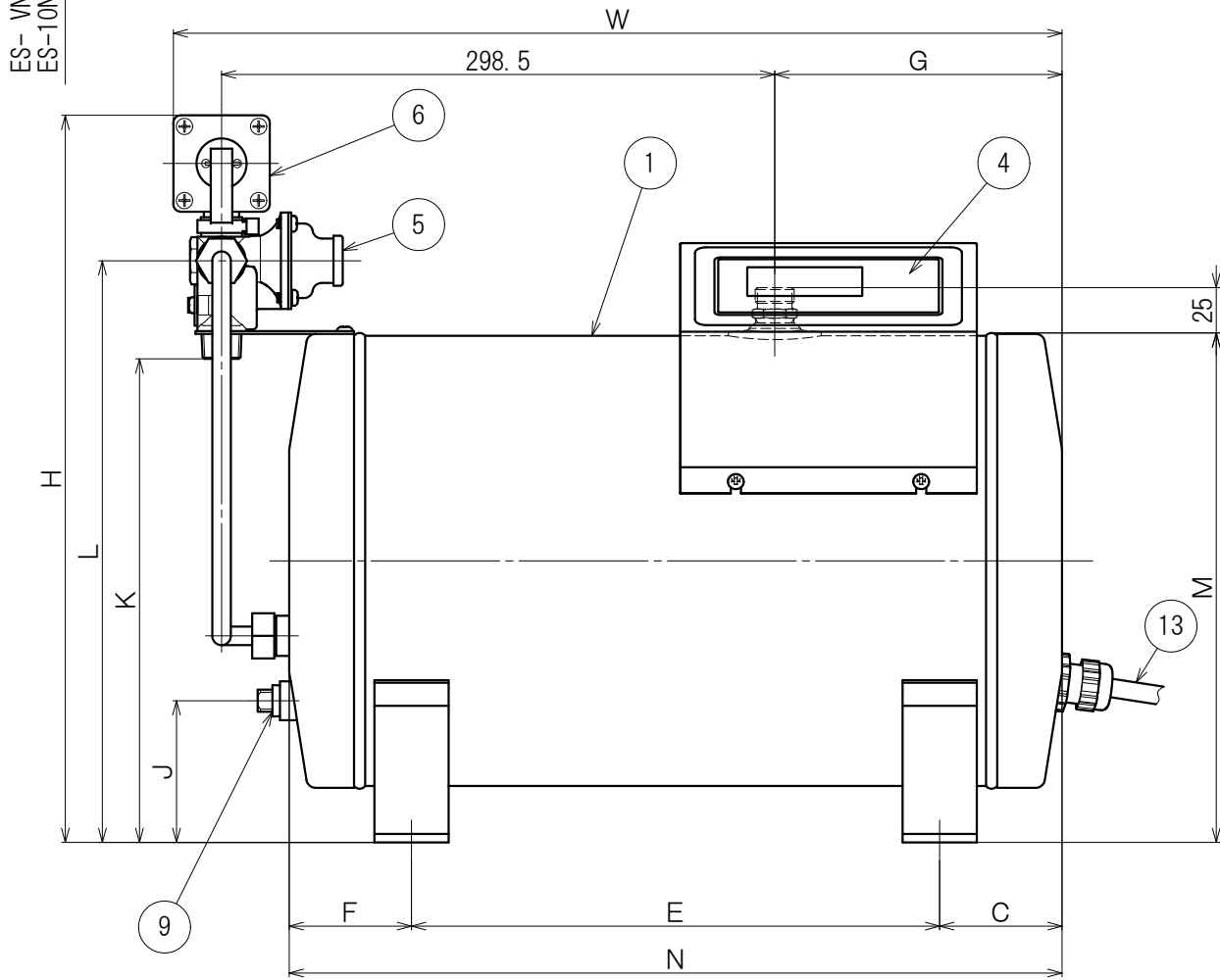
正面図
