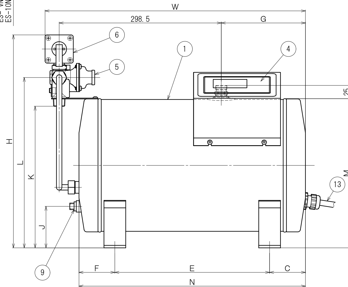
正面図
