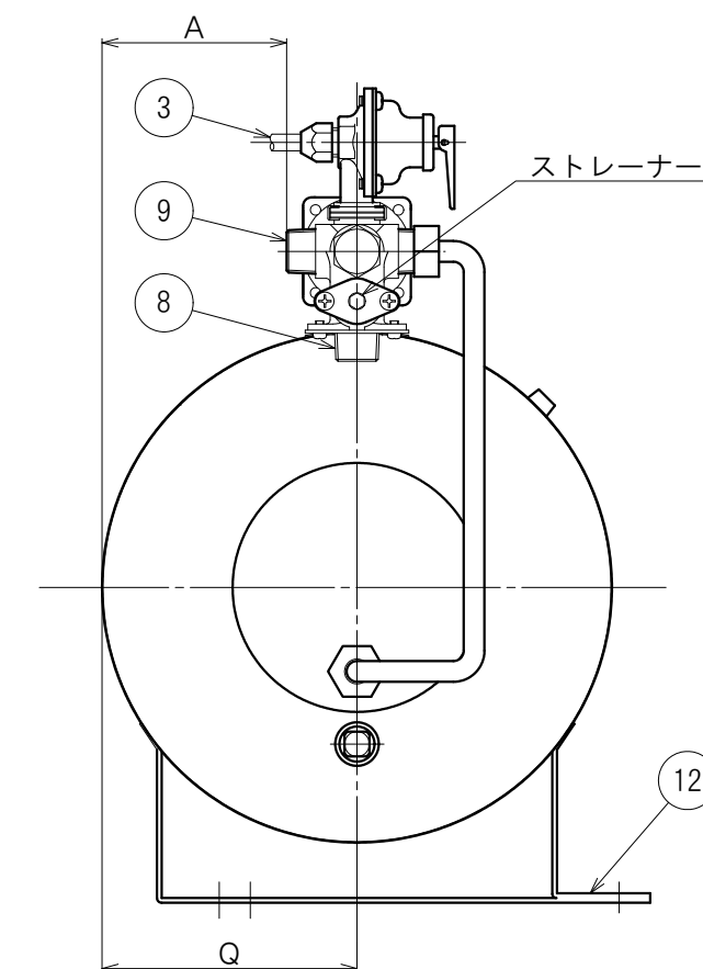
左側面図
