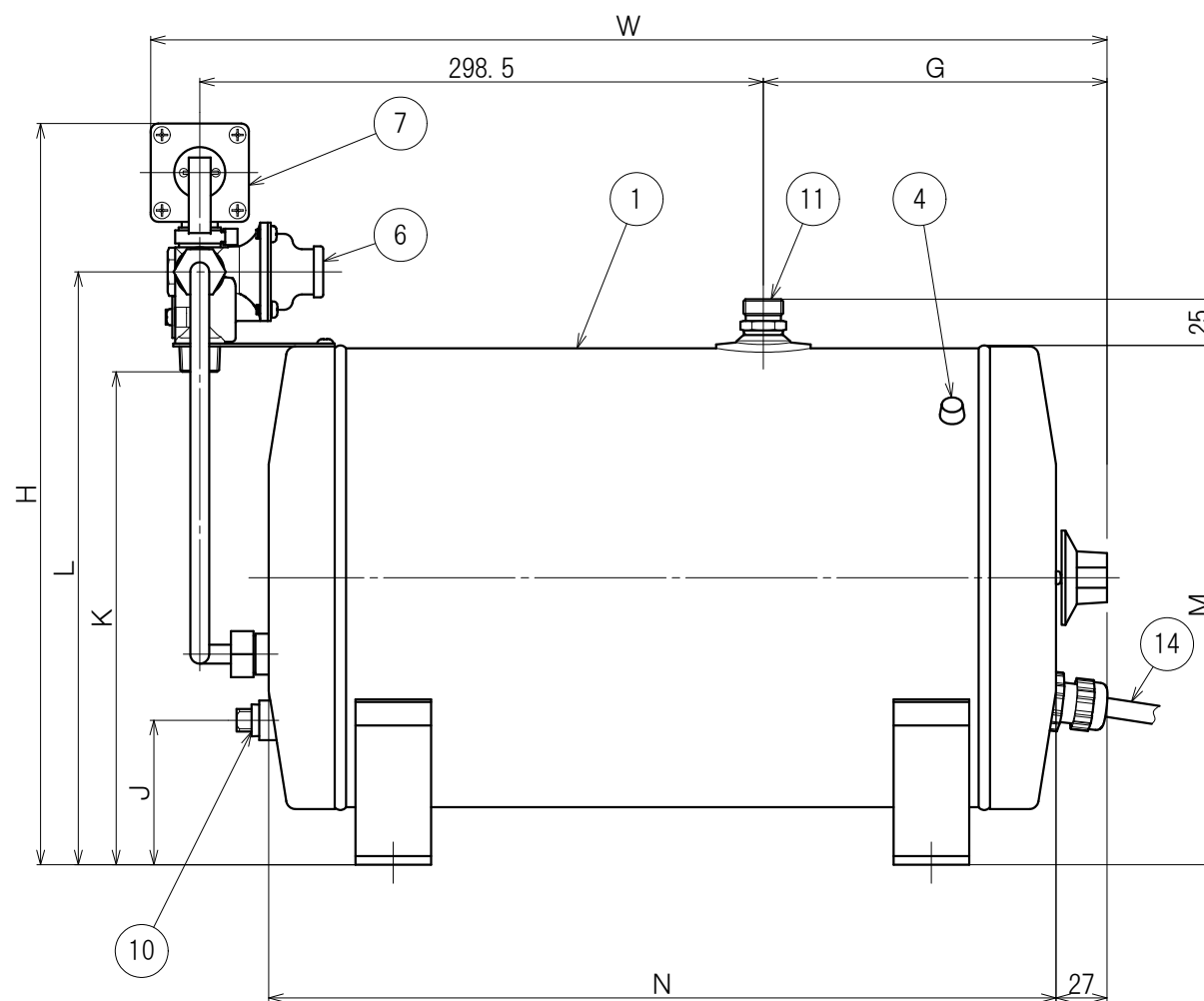
正面図
