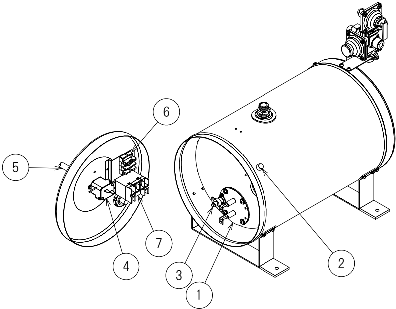
部品配置図
