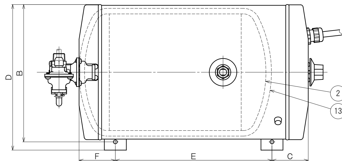
平面図
