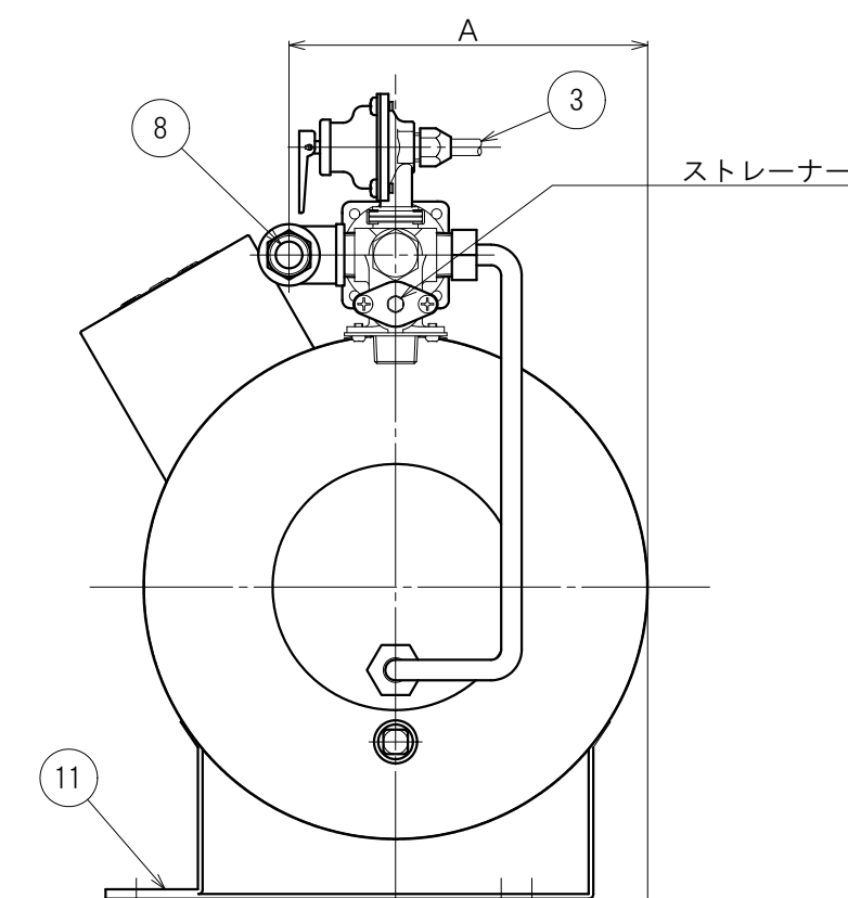
右側面図
