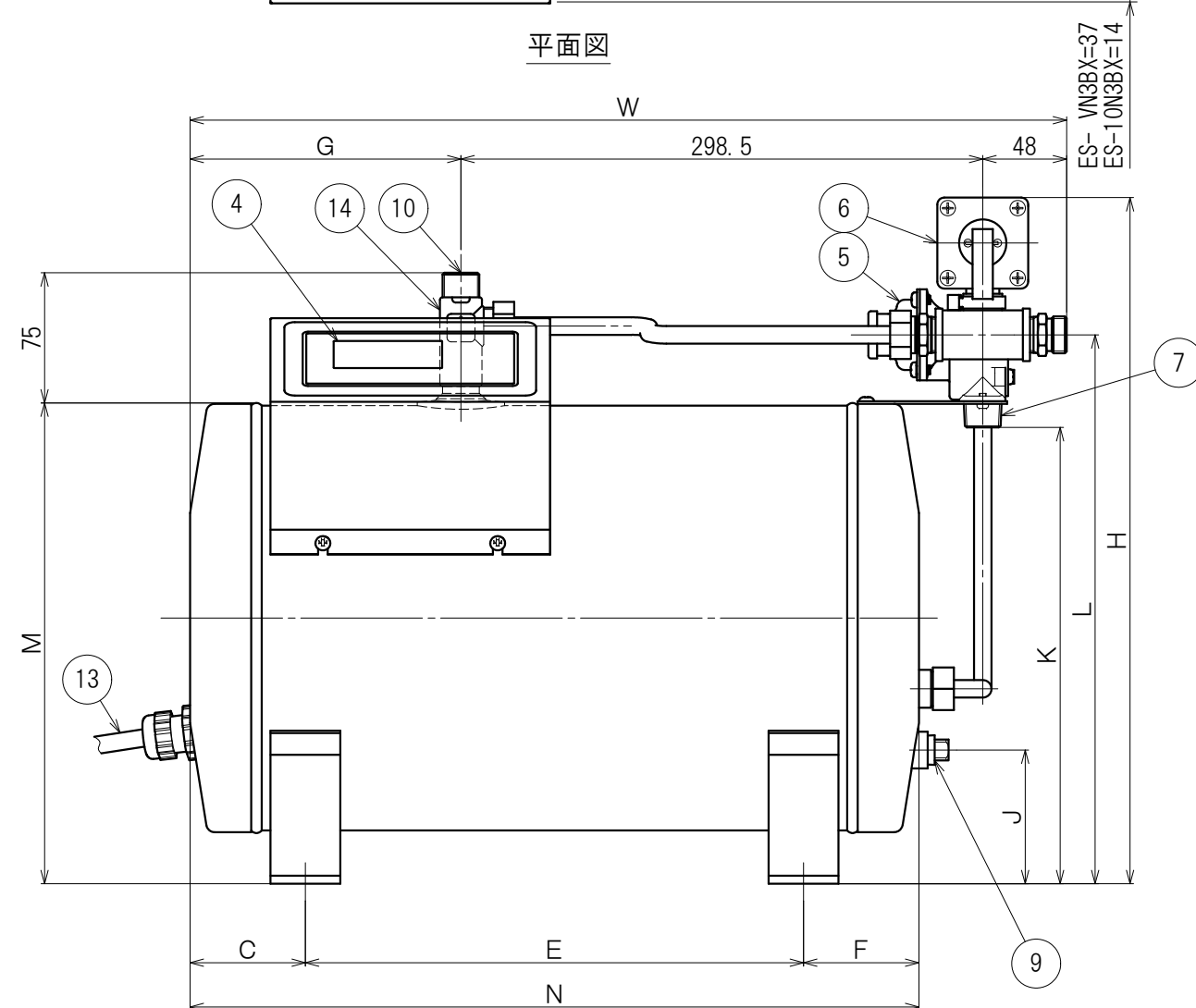
正面図
