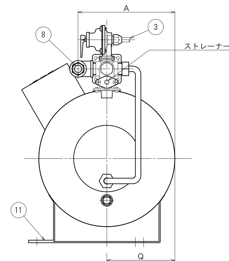
右側面図
