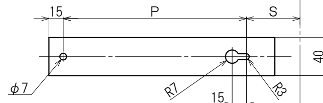
右側面図
