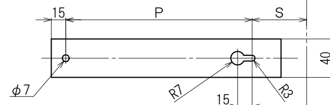
右側面図
