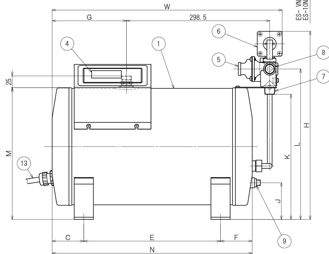
正面図
