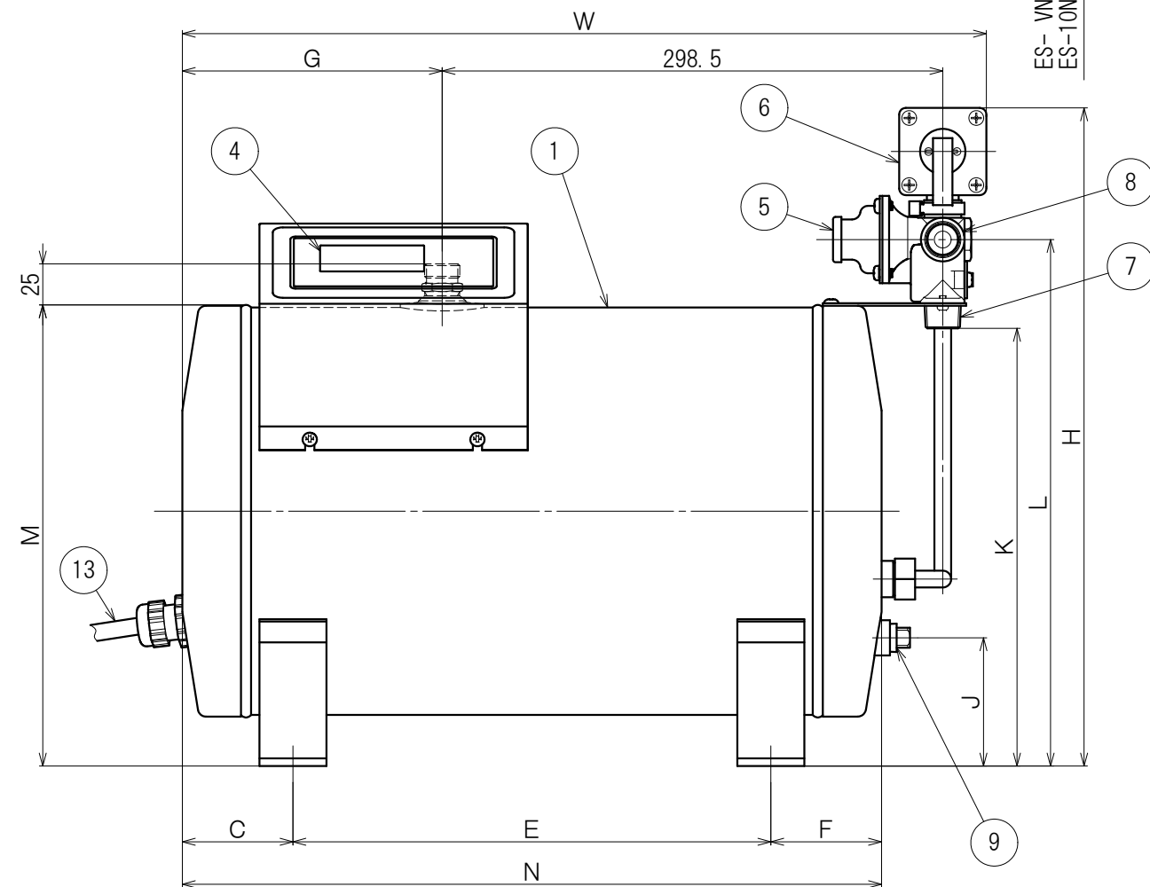
正面図
