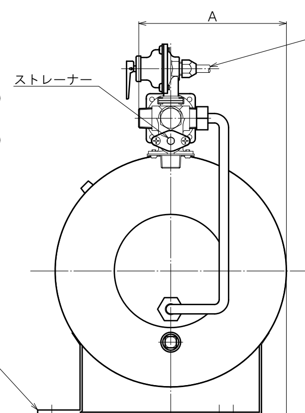
右側面図
