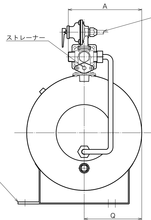
右側面図
