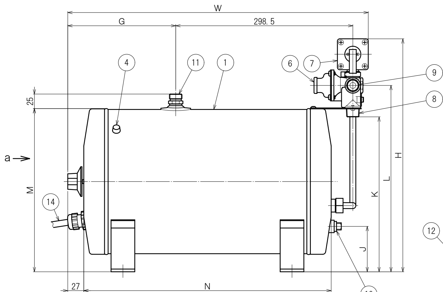
正面図
