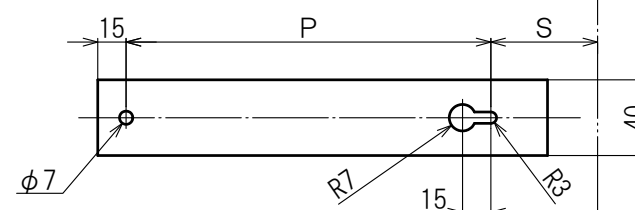
右側面図
