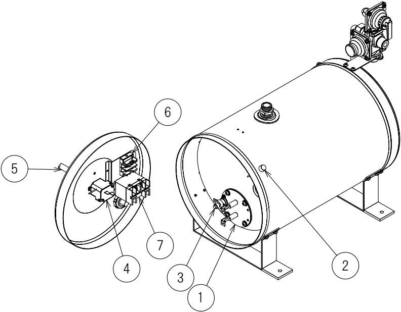
部品配置図
