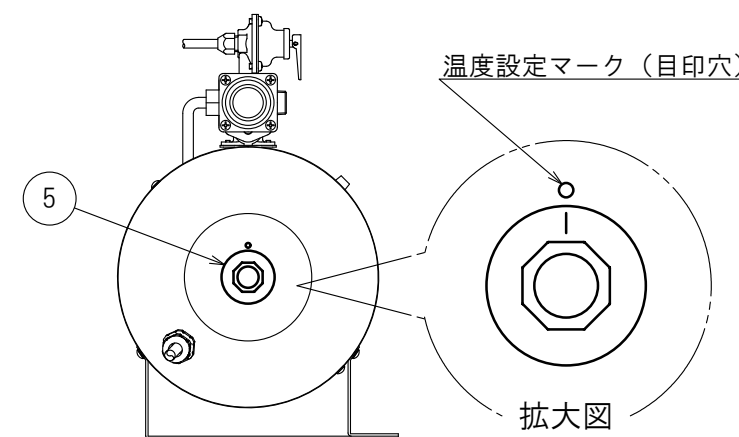
a 矢視図
