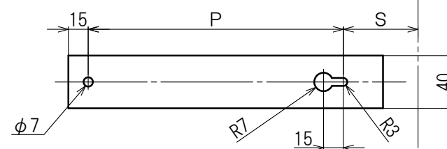
右側面図
