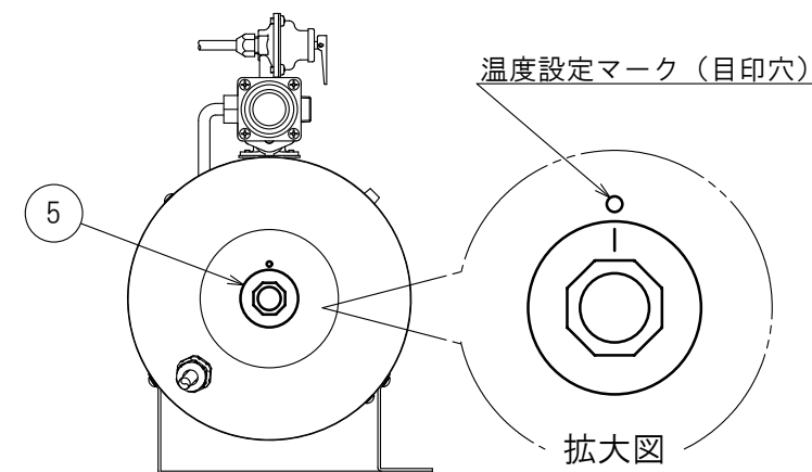
a 矢視図
