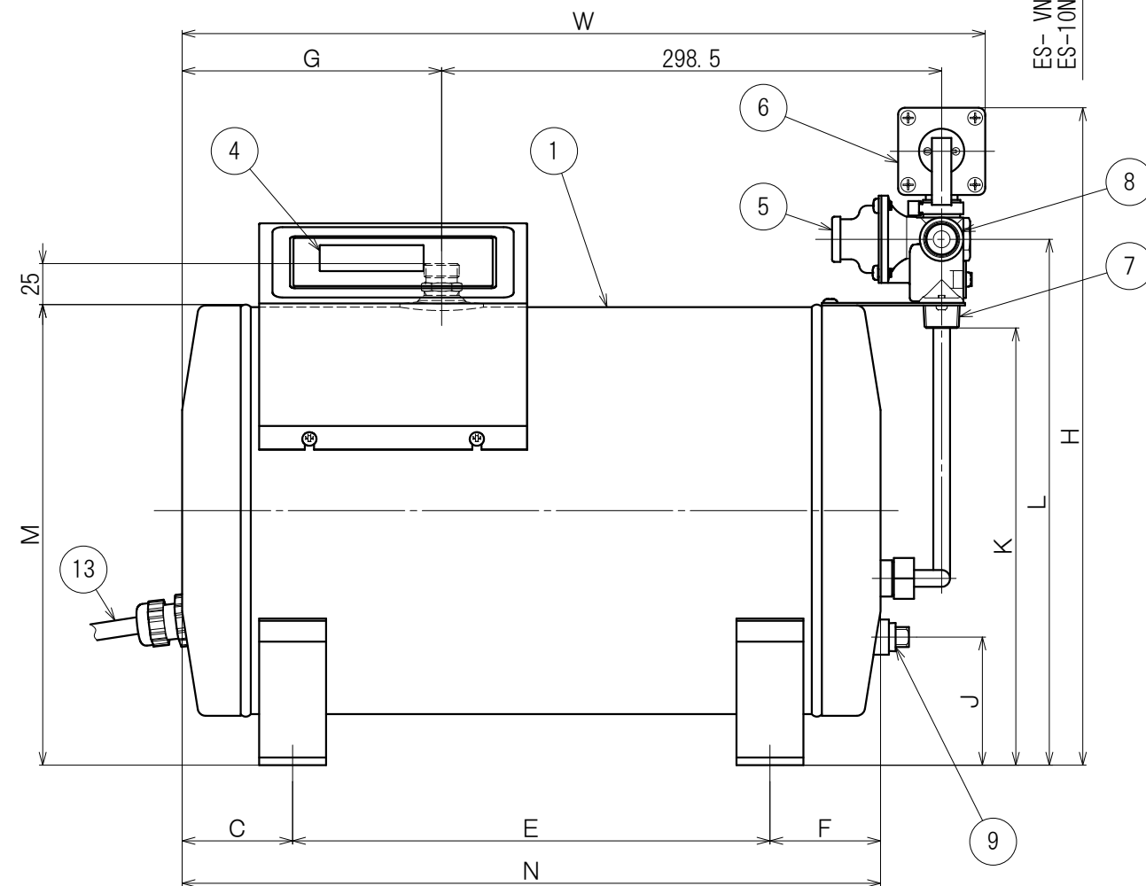
正面図
