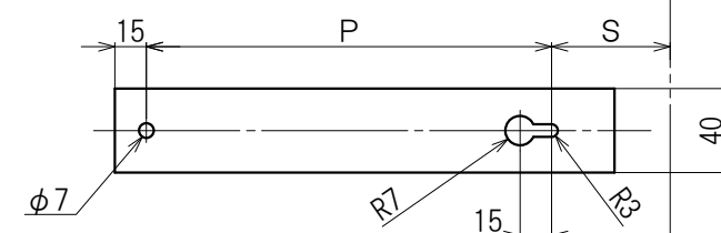
右側面図
