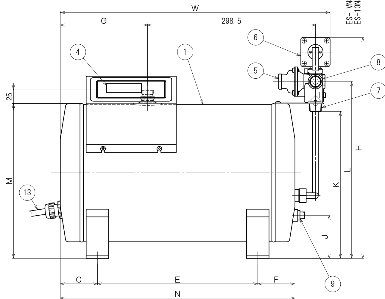
正面図
