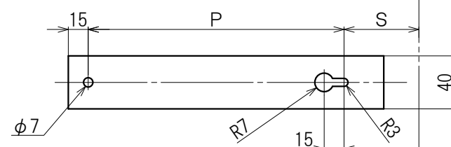
右側面図
