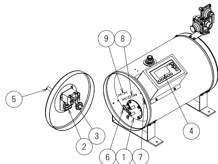
部品配置図 図はES-10N3B(2)
