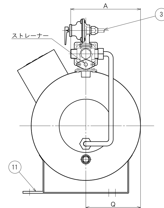
右側面図
