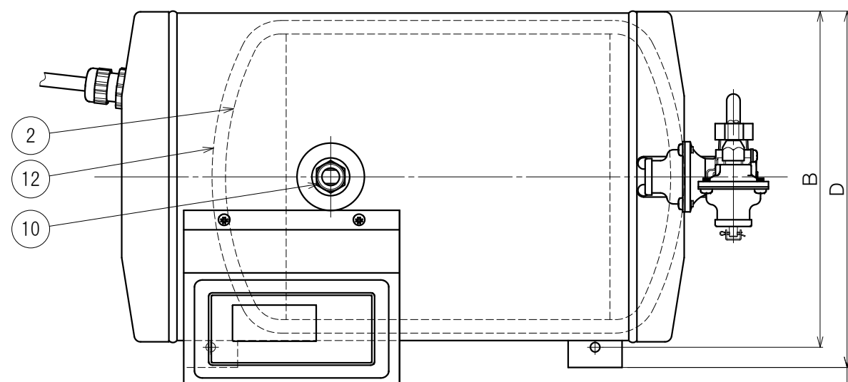
平面図
