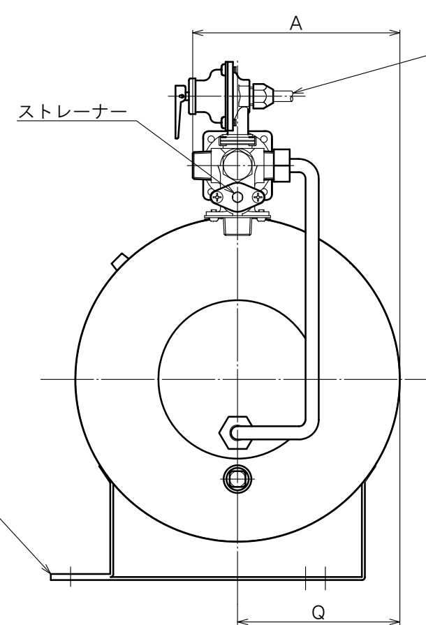
右側面図
