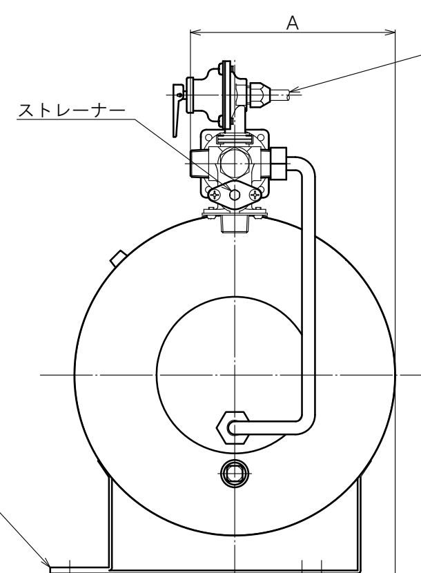
右側面図
