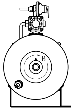
A矢視図
