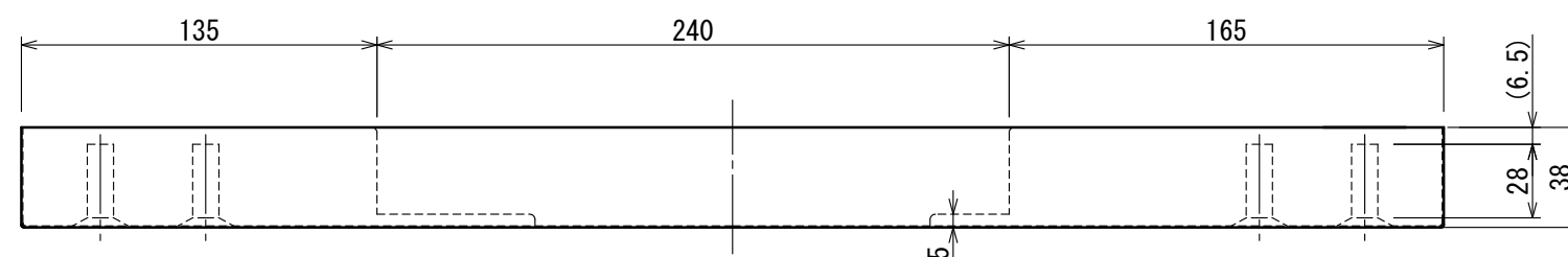
正面図
