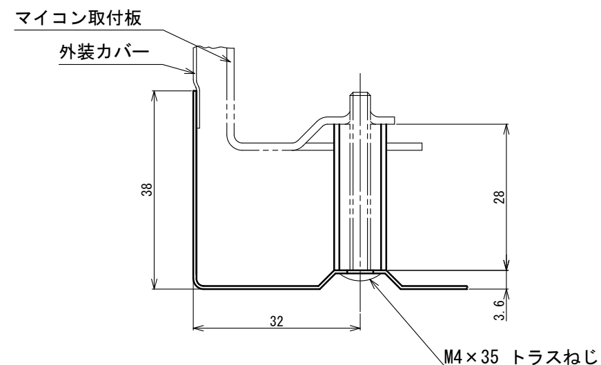
A-A断面図
