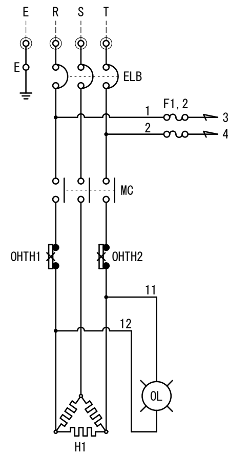
主回路 3φ200V 3. 1～5kW
