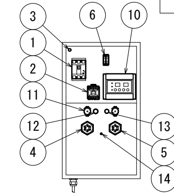
電装ケース部品配置図 7.1kW~9kWの場合
