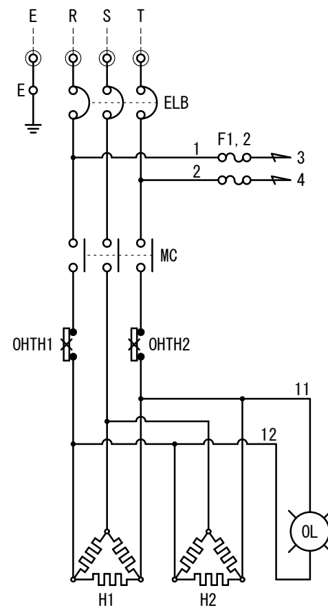
主回路 3φ200V 7. 1～9kW
