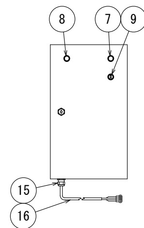
電装ケース部品配置図 3.1kW~5kWの場合
