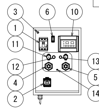
電装ケース部品配置図 7.1kW~9kWの場合
