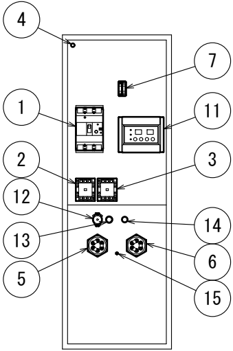
電装ケース部品配置図
