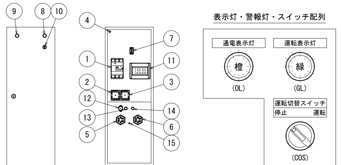
電装ケース部品配置図
