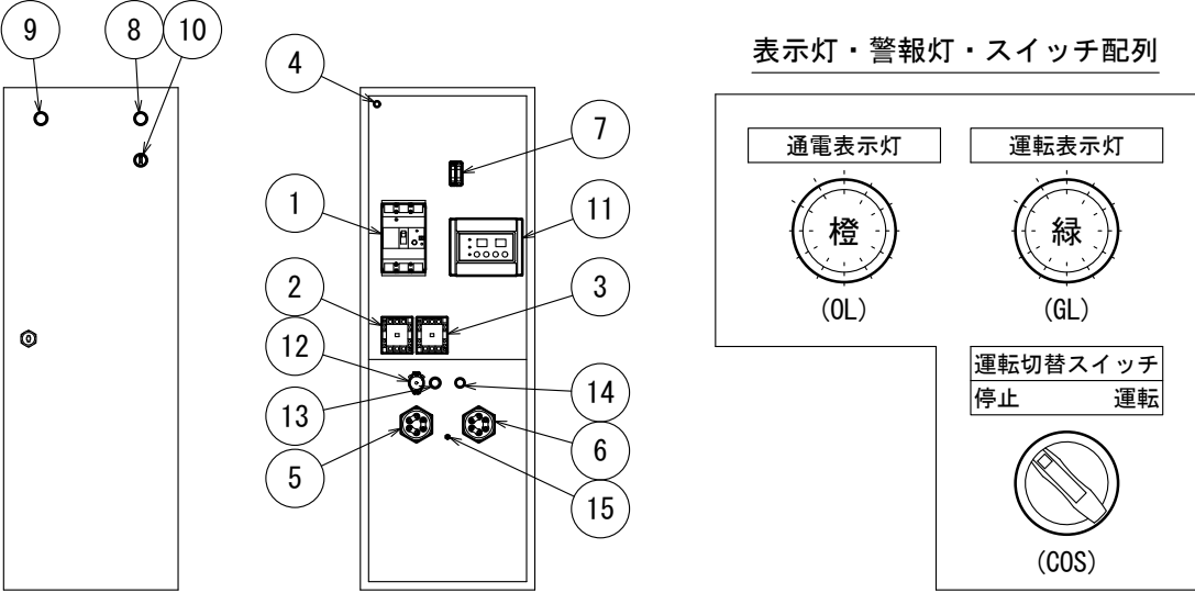
電装ケース部品配置図
