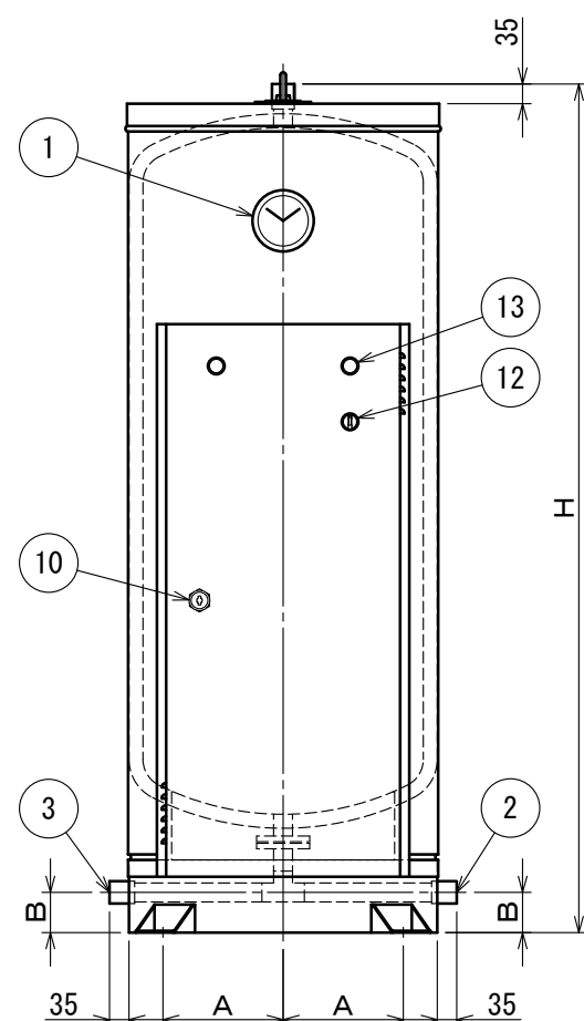
正面図
