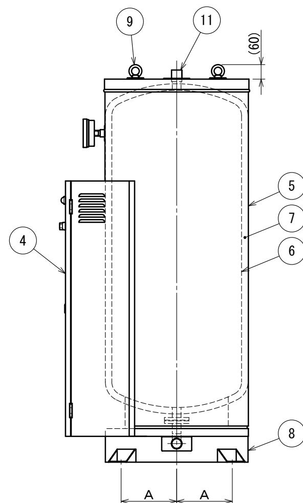
右側面図
