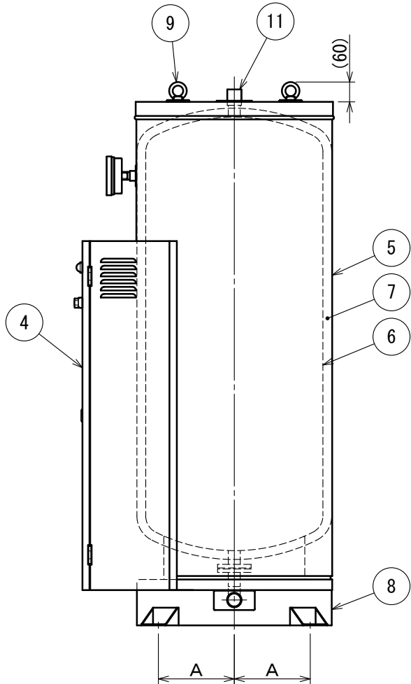
右側面図
