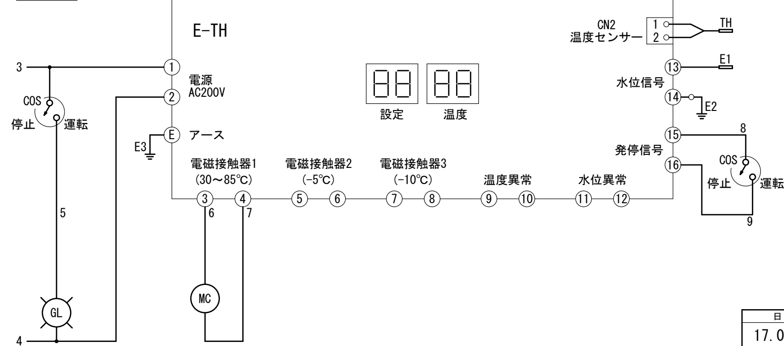
操作回路
