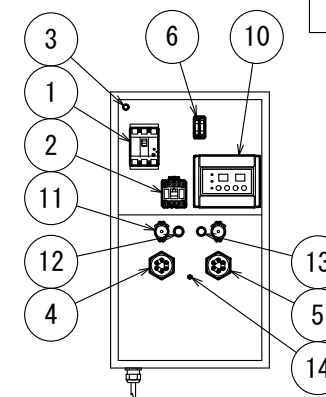
電装ケース部品配置図 7.1kW~9kWの場合
