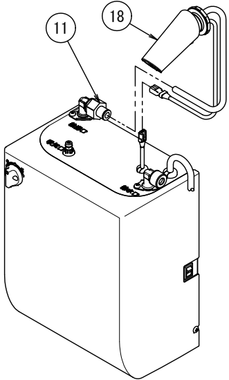
アイソメ図《自動水栓組立》
