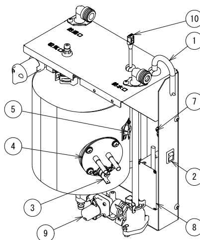
部品配置図 ESWM3ASK
