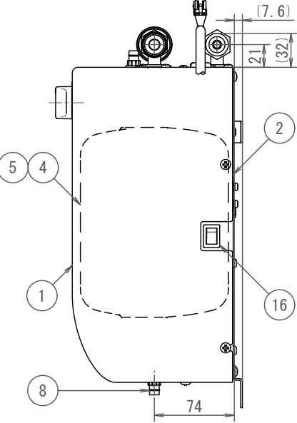
固定ねじ穴位置図
