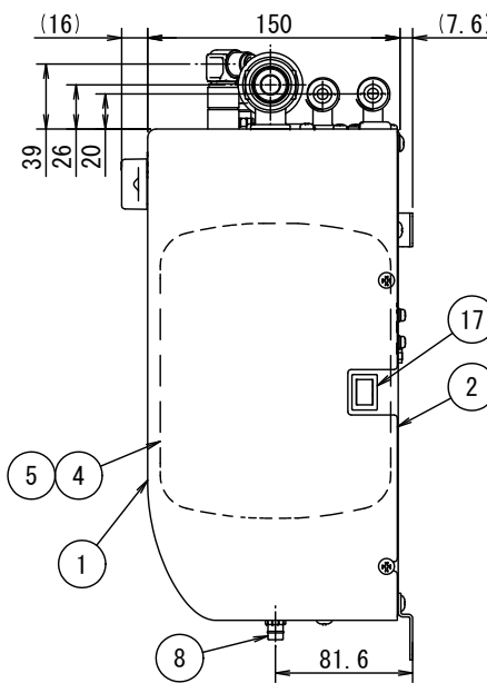
【右側面図】
