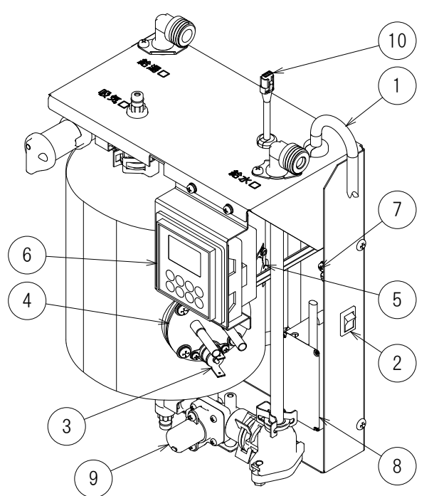
部品配置図 ESWM3TSS
