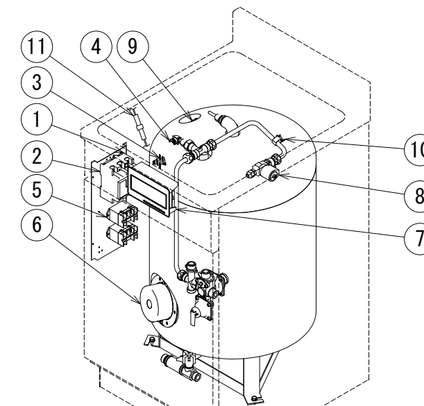
部品配置図
