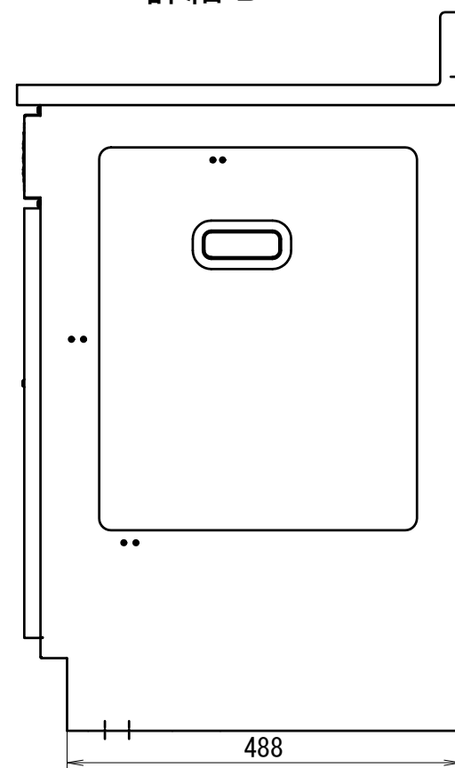
右側面図
